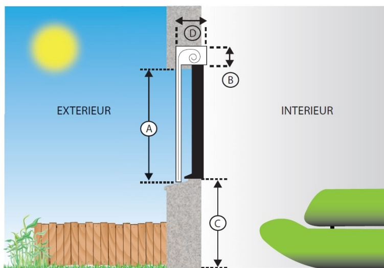
COFFRE SOUS LINTEAU (TRADITIONNEL)
